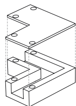
342 accessorio blocco di raccordo angolare a 90° con copertura connecting block 90° corner with cover
