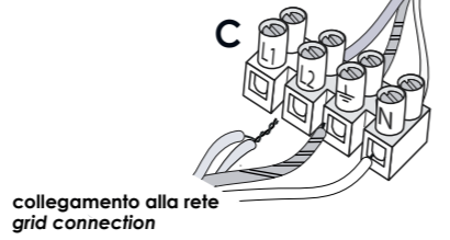
collegamento alla rete grid connection
