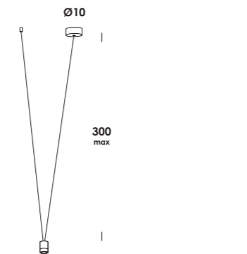
m.t.o. 10/so dim 3,5w 350mA 330lm 3000K - 230V fornito con driver e modulo led integrato di classe A+ luminaire contains driver and led A+
